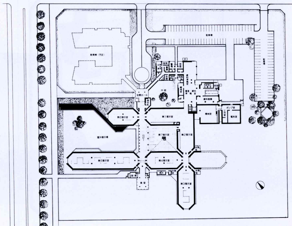
1階平面図
