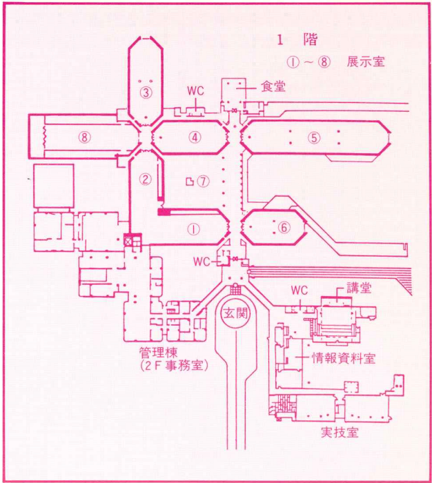
千葉県立美術館 平面図
