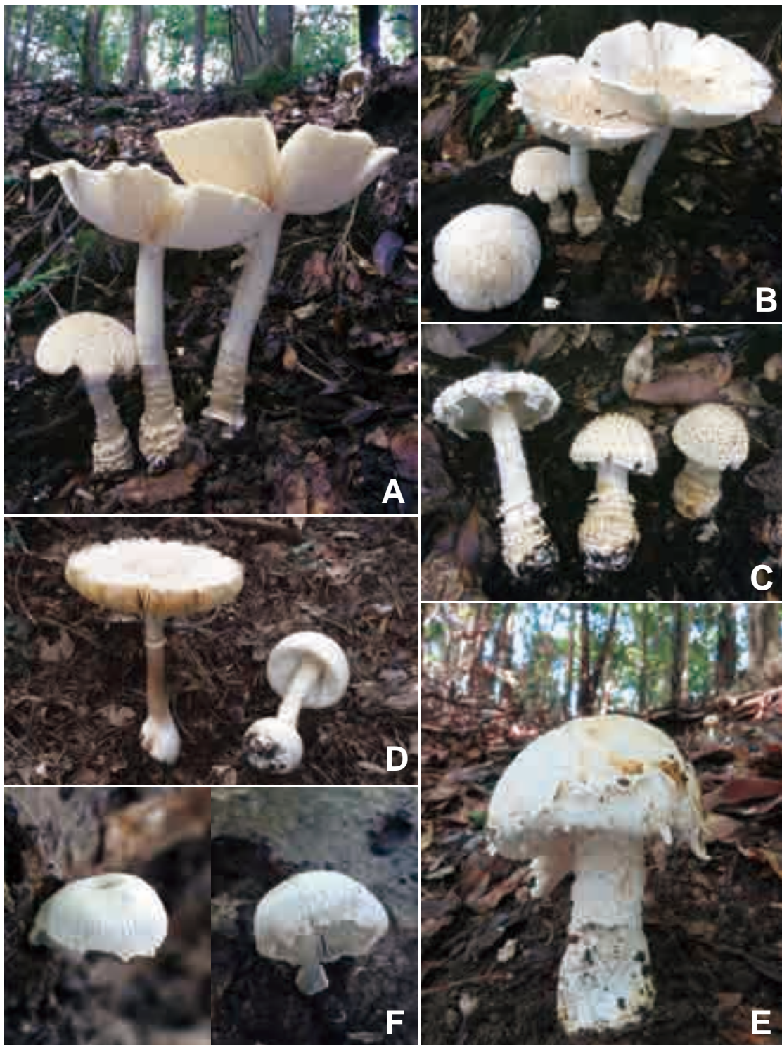
シイ・カシ林の大形担子菌類. A-C: 15) シロオビテングタケ Amanita concentrica , 2000年10月2日, 荒樫沢, CBM-FB-24901 Holotype. D: 20) カブラテングタケ Amanita gymnopus , 2012年7月31日, 檜の木台, CBM-FB-31557. E: 24) シロテングタケ Amanita neo-ovoidea , 2015年9月11日, 荒樫沢, CBM-FB-40806. F: 75) ヤコウタケ Mycena chlorophos , 1989年7月22日, CBM-FB-2345.
