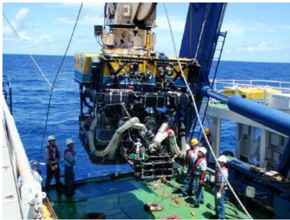
無人探査機「ハイパードルフィン」。「なつしま」船尾から出し入れされます。
